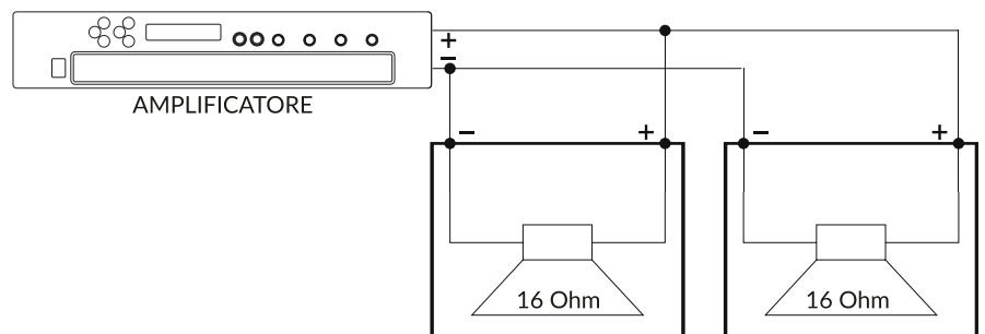
IMPEDENZA TOTALE 8 OHM
